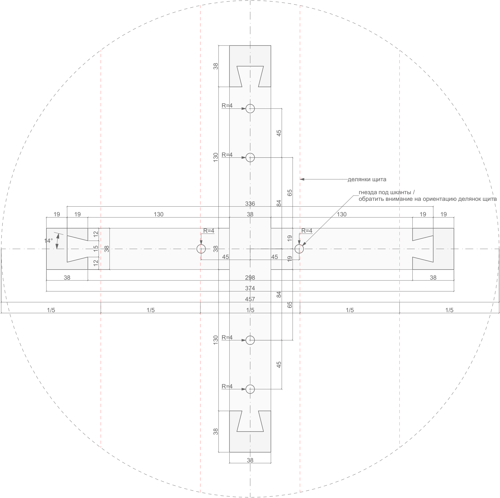
Gustav Stickley. No 603 Tabouret разрез 2-2 / М 1:2
