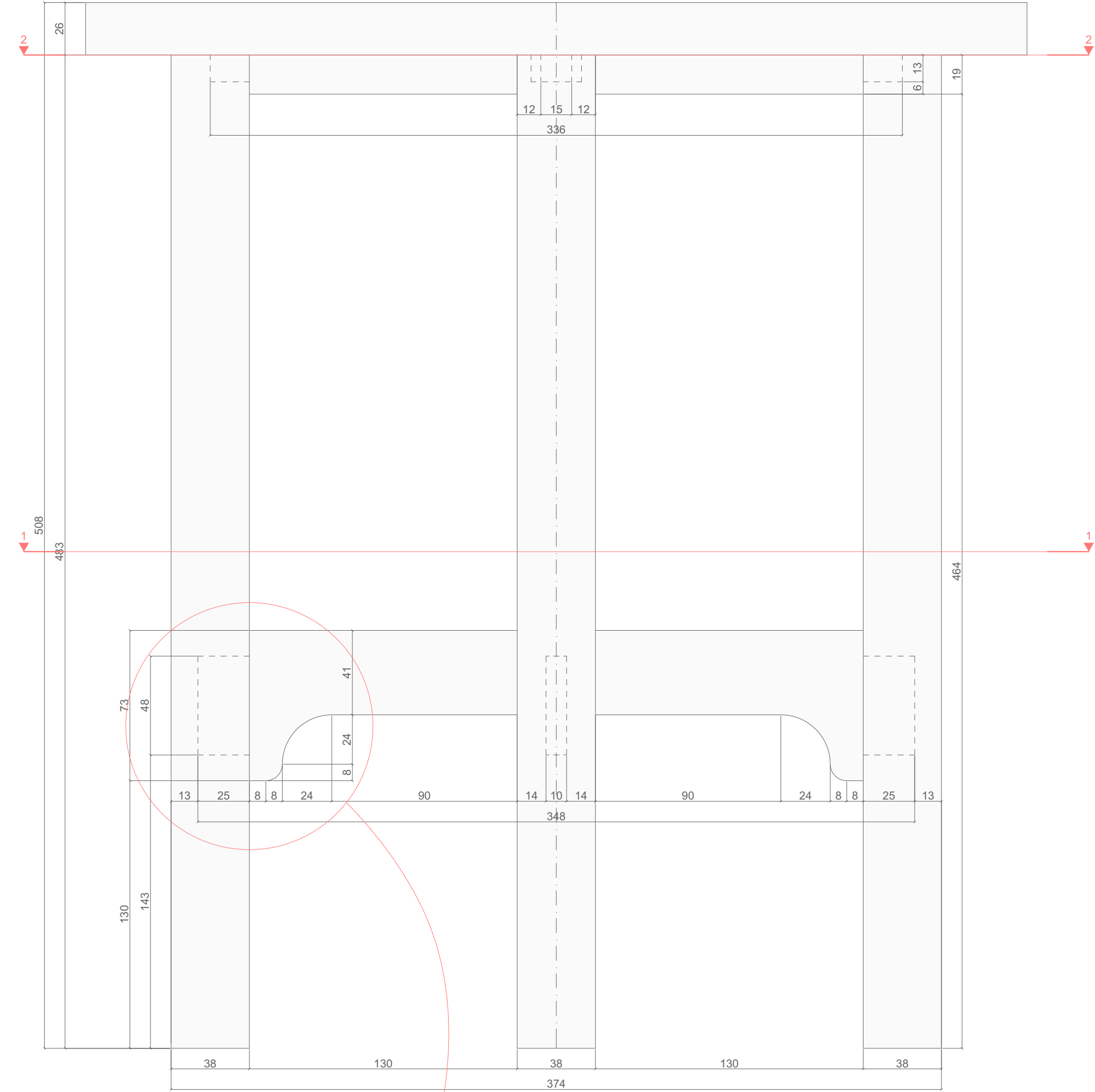
деталь / М 1:1
