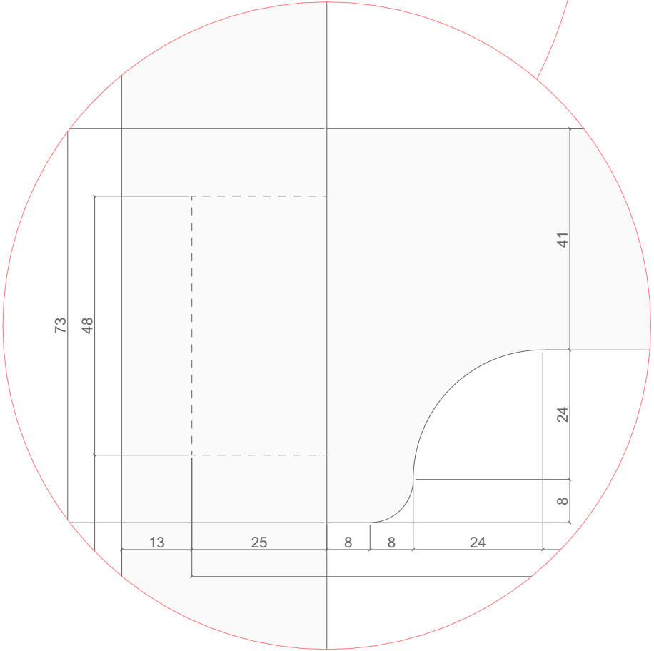
деталь / М 1:1
