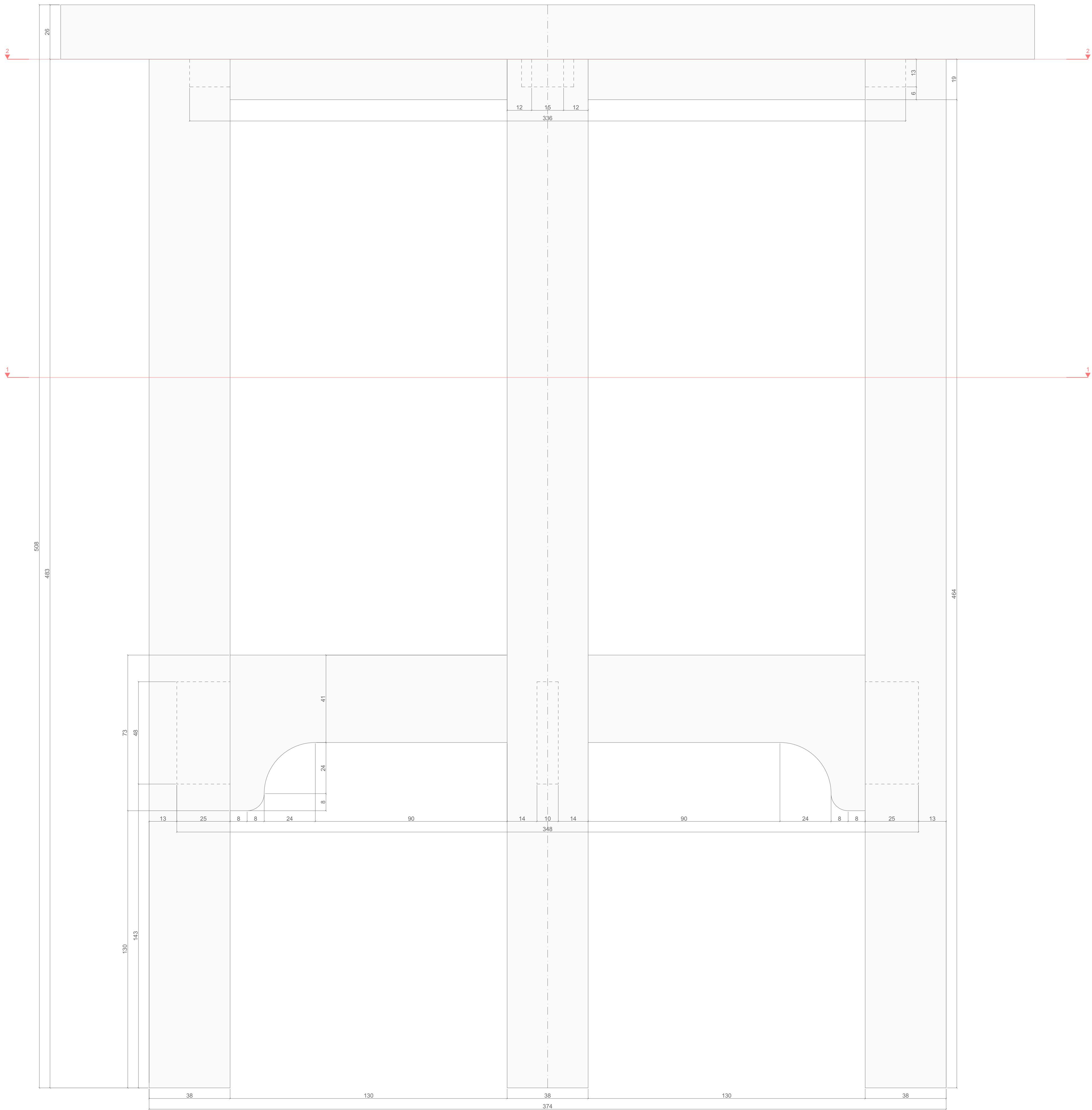
Gustav Stickley, No 603 Tabouret Фронтальный вид / M 1:1
